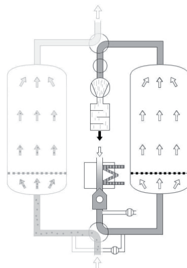
Verhittingsfase
