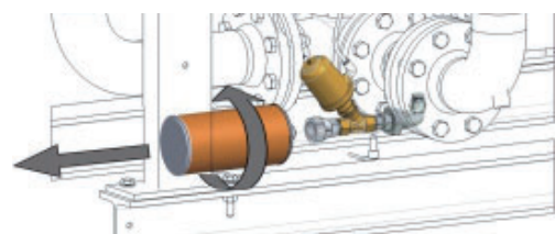
Geluiddemper losdraaien
